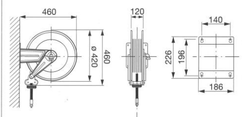
Dimensioner - ydermål (mm) Serie 430 åben ABS fast
