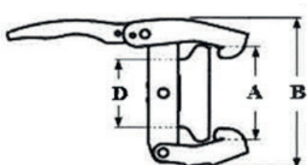
Måltegning
