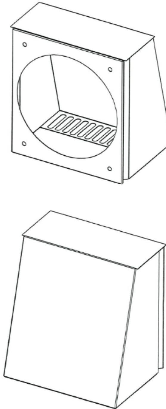
Yderdæksel m/bredt lamelspjæld til ZEPHYR, varenr. TWHEATQ066
